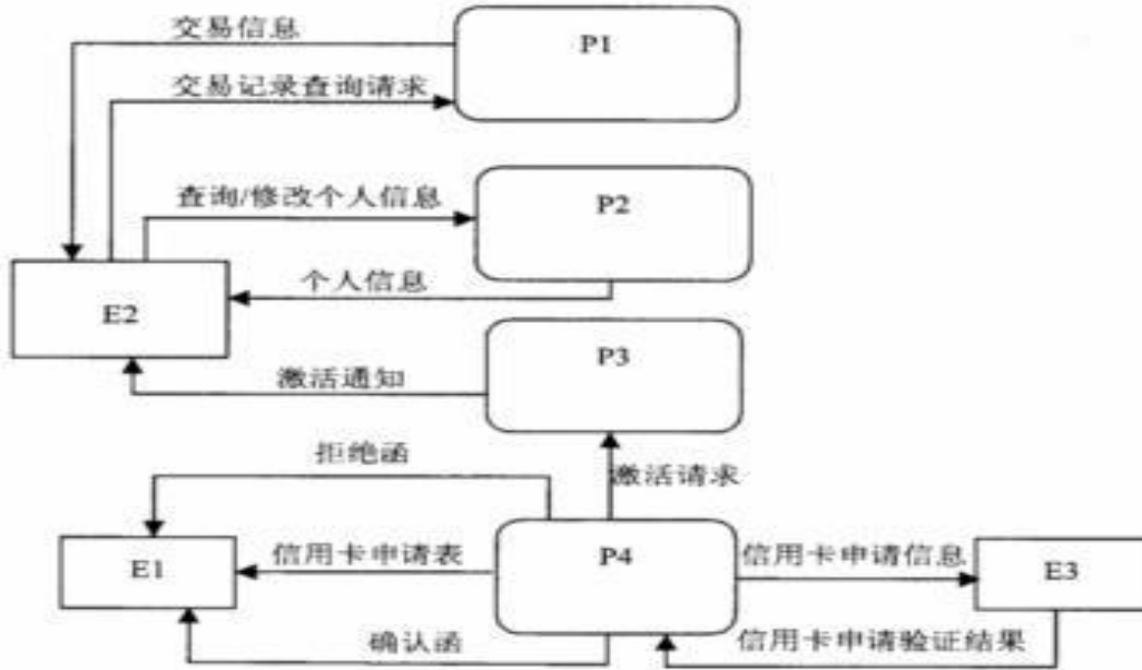
图 1-2 0 层数据流图
