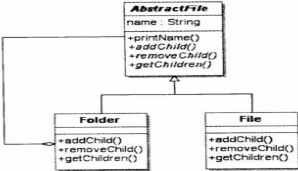
图 5-1 类图
