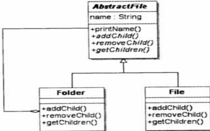
图 5-1 类图
