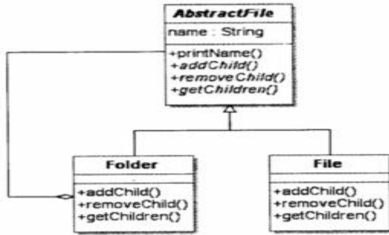
图 6-1 类图
